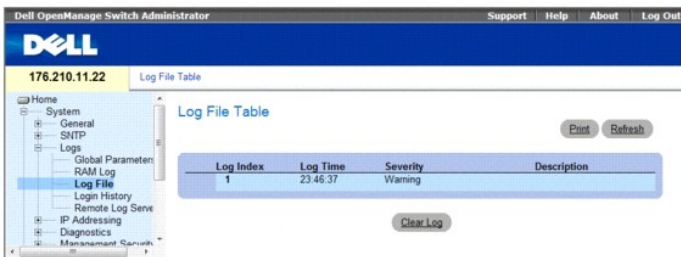
Рис. 6-17. Таблица файла журнала
