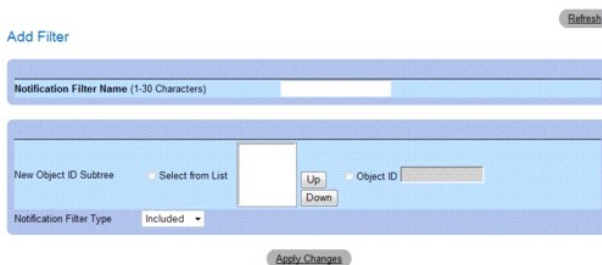
Рис. 6-96. Add Filter (Добавление фильтра)
