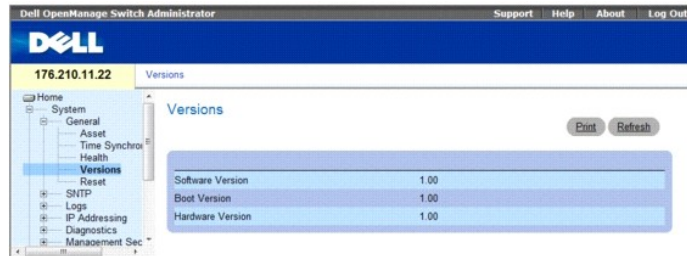
Рис. 6-5. Версии
