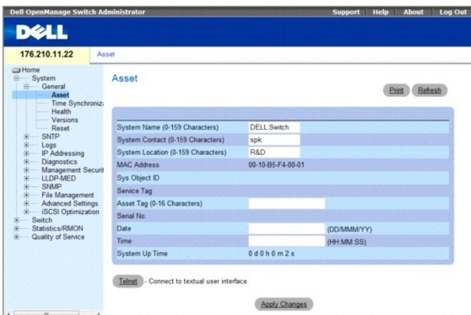
Рис. 6-2. Ресурсы
