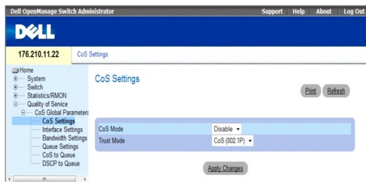
Рис. 9-1. Параметры CoS
