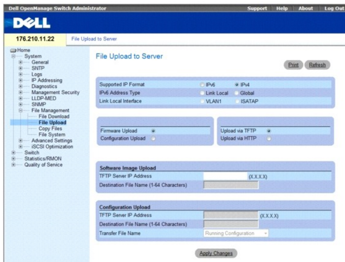
Рис. 6-101. File Upload to Server (Передача файлов на сервер)
